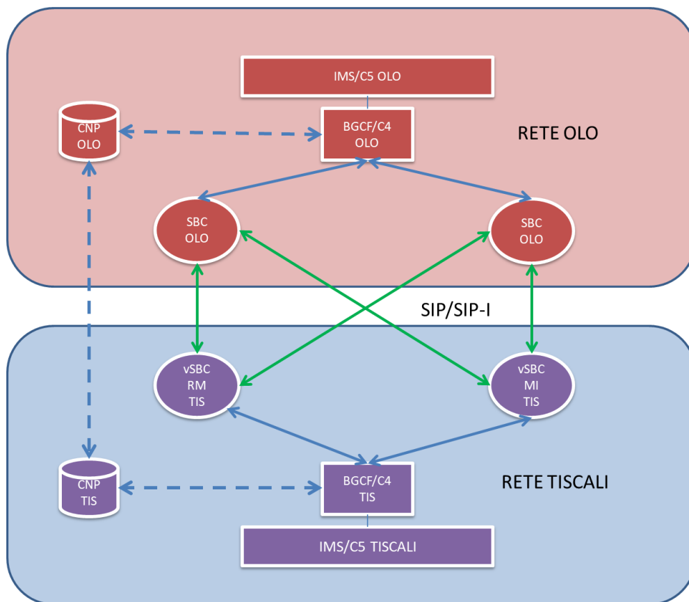
Figura 1: Modello di interconnessione IP con Pdl attuali
