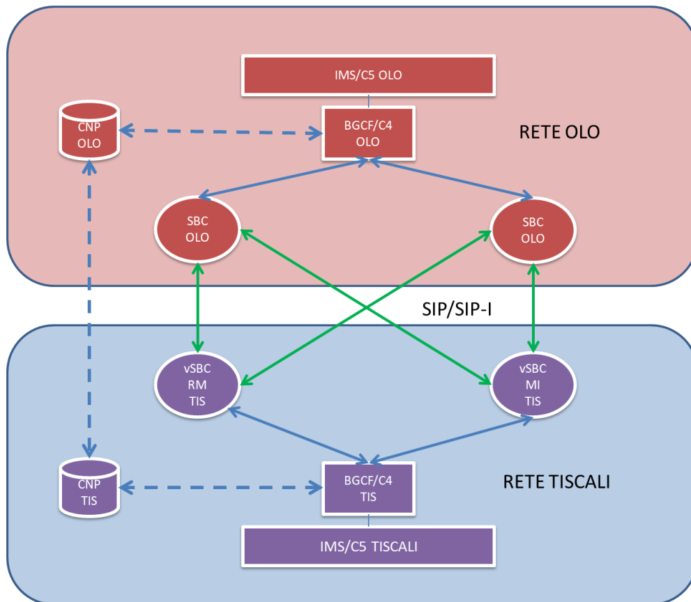
Figura 1: Modello di interconnessione IP con PDI attuali
